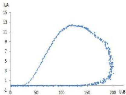
Рис. 4. ВАХ нагрева образца из стали 20 в водном растворе \text{NH}_4\text{Cl} ( c = 3 моль/л). Емкость батареи конденсаторов 0 мкФ.
