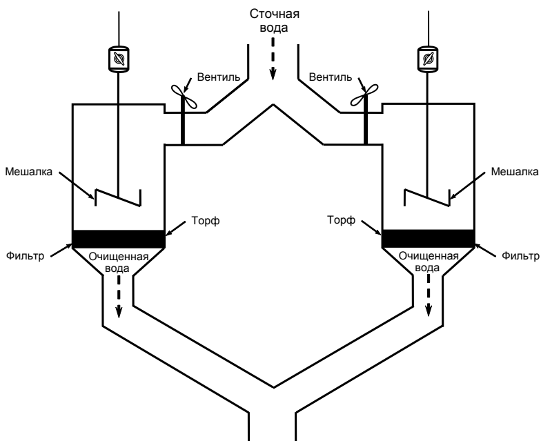
Рисунок 2 – Принципиальная технологическая схема сорбционной очистки сточных вод от ионов тяжелых металлов
