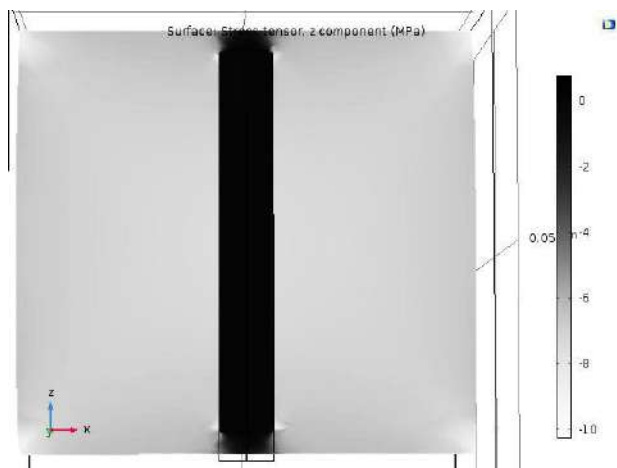
Рисунок 3. Изополе напряжений по оси Z
