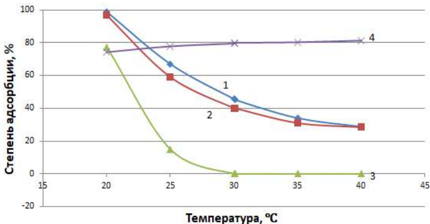
Рисунок 2 – Зависимость степени адсорбции тиомочевины от температуры процесса при разных модификаторах кремнегеля
