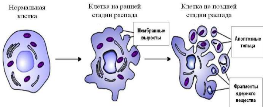
Рисунок 1 – Схема программируемого клеточного распада (апоптоза).
