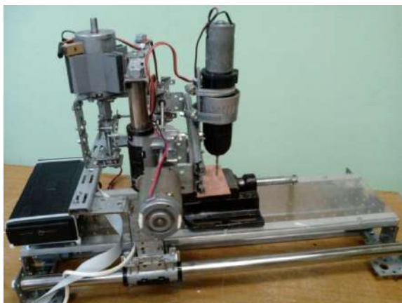
Внешний вид собранного станка
