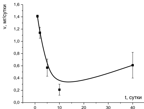
Рис. 2. Зависимость скорости коррозии от времени выдержки.
