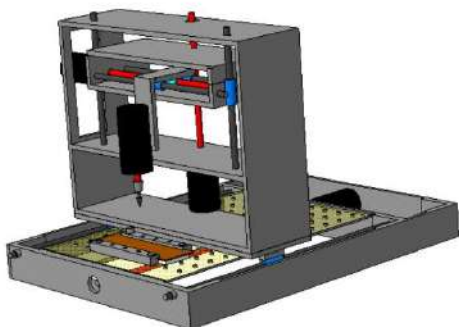
Механическая компоновка учебного малогабаритного фрезерно-сверлильного 2D станка с ЧПУ
