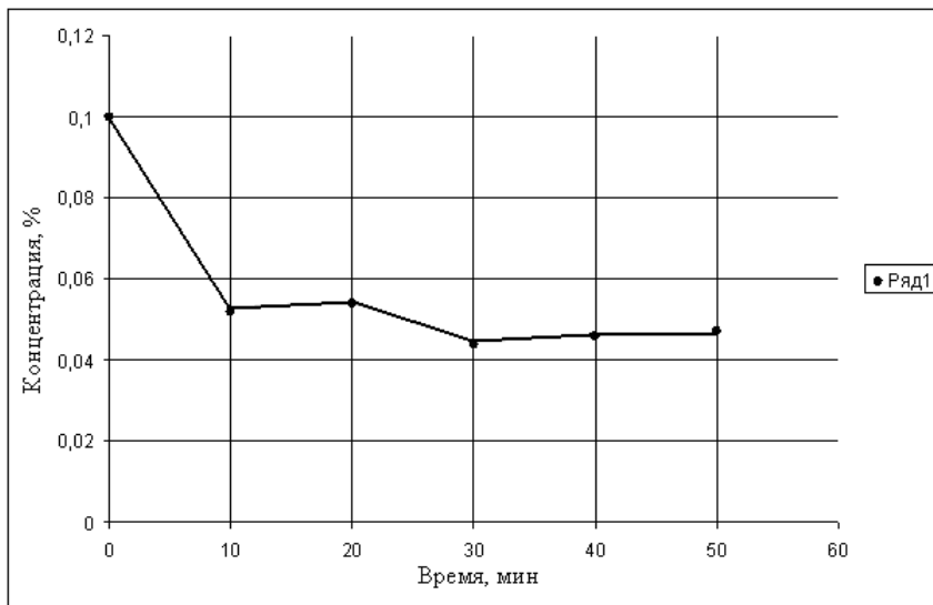
Рисунок 3 – Кинетическая кривая адсорбции индигокармина
