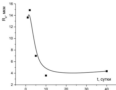
Рис. 3. График зависимости шероховатости поверхности от времени выдержки.
