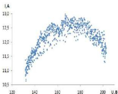
Рис. 3. ВАХ нагрева образца из стали 20 в водном растворе \text{NH}_4\text{Cl} ( c = 3 моль/л). Емкость батареи конденсаторов 2600 мкФ.
