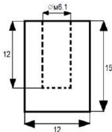
Рис. 1. Чертёж образца для коррозионных исследований. Размеры на рисунке указаны в мм.
